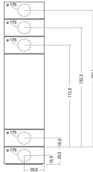
Rauchrohrabgang (oben)
