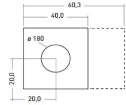
Rauchrohrabgang (oben)
