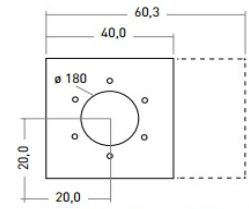
Frischluftzufuhr (unten)
