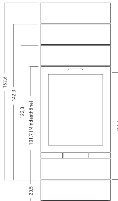
Frontansicht
