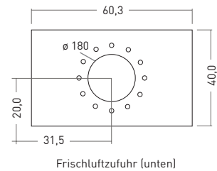
Frischluftzufuhr (unten)
