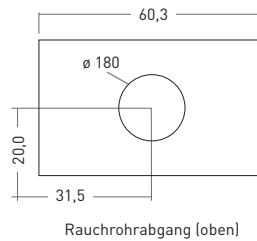
Rauchrohrabgang (oben)
