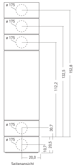
Seitenansicht
